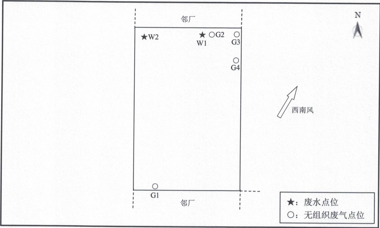
测点示意图
